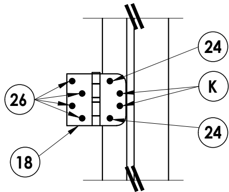
HINGE JAMB
